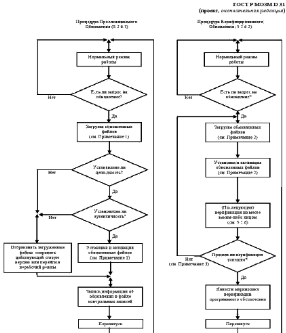
Рисунок 1 - Процедуры обновления программного обеспечения.
